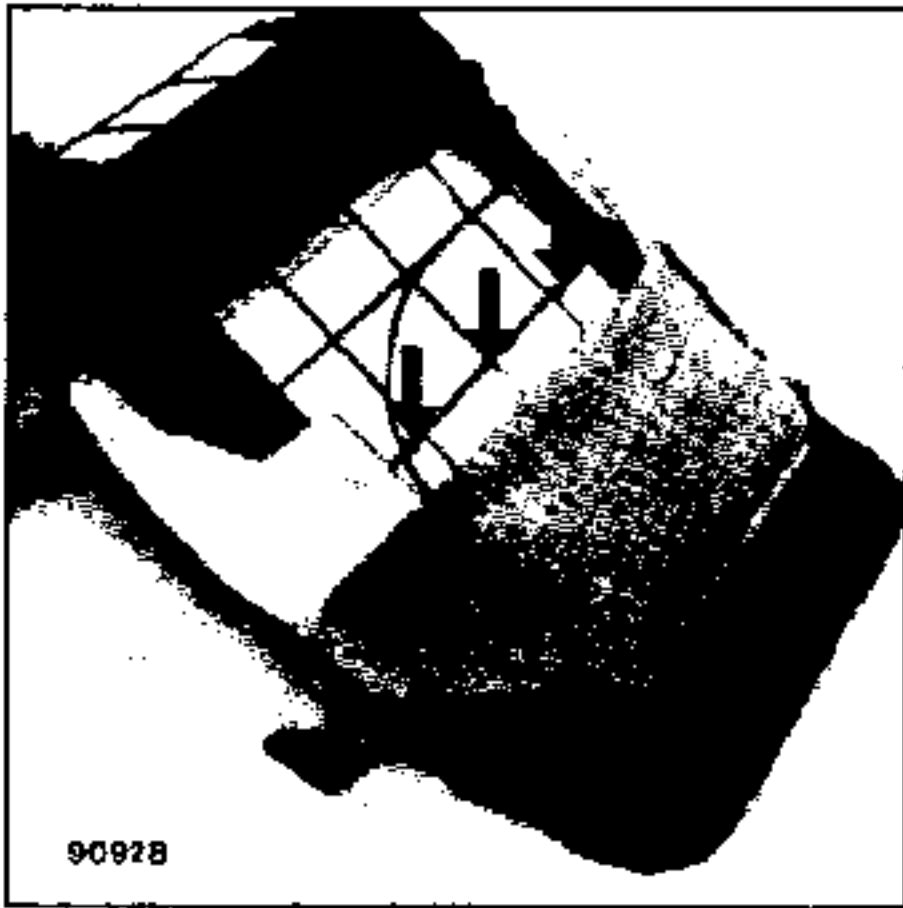
Die drei mittleren Klammern durchschneiden, und den Sitzbezug umlegen, um an das andere Ende des Seilzuges zu gelangen.
